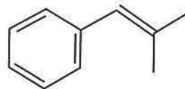
1-fenil-2-metilprop-1-eno
